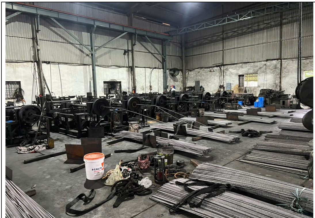
Hệ thống cán ren bán tự động
